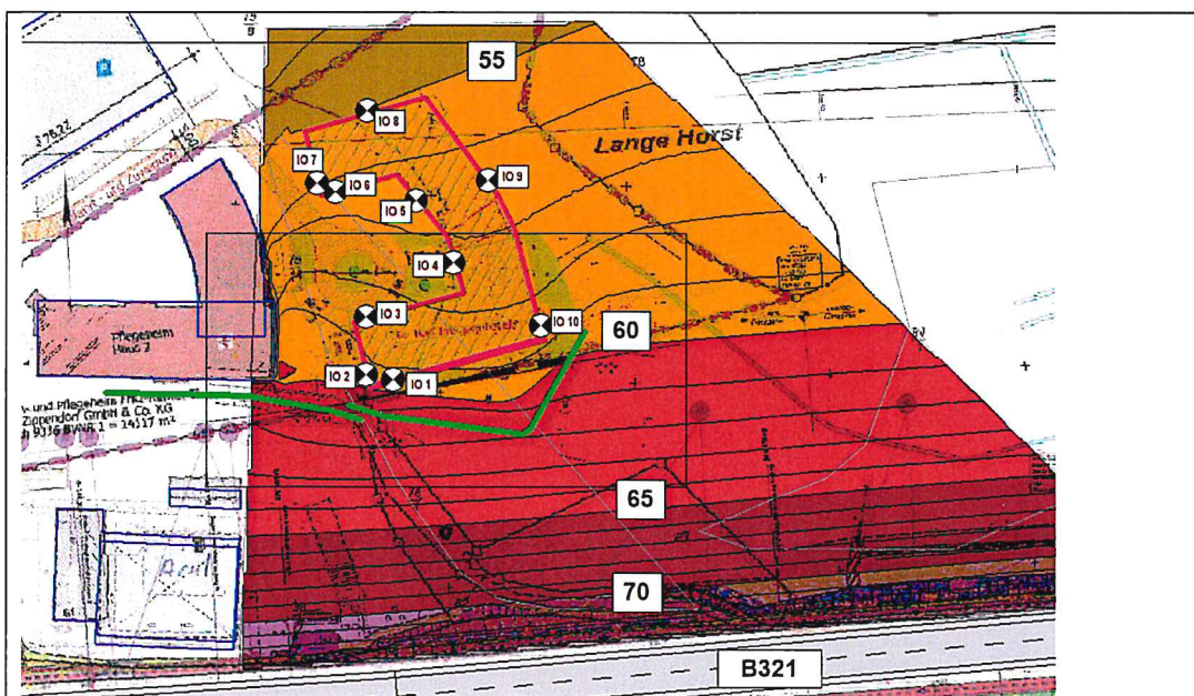
Abb. 4: Lärmpegelkarte, Bsp. Beurteilungspegel Tageszeit mit Wall-H = 5,0 m im OG
